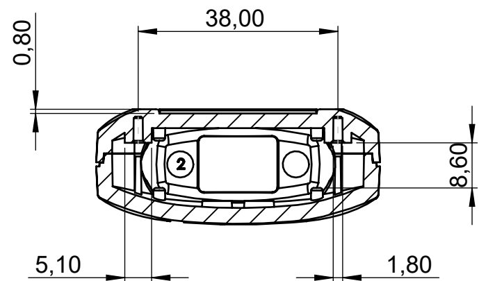
Schnitt A-A
