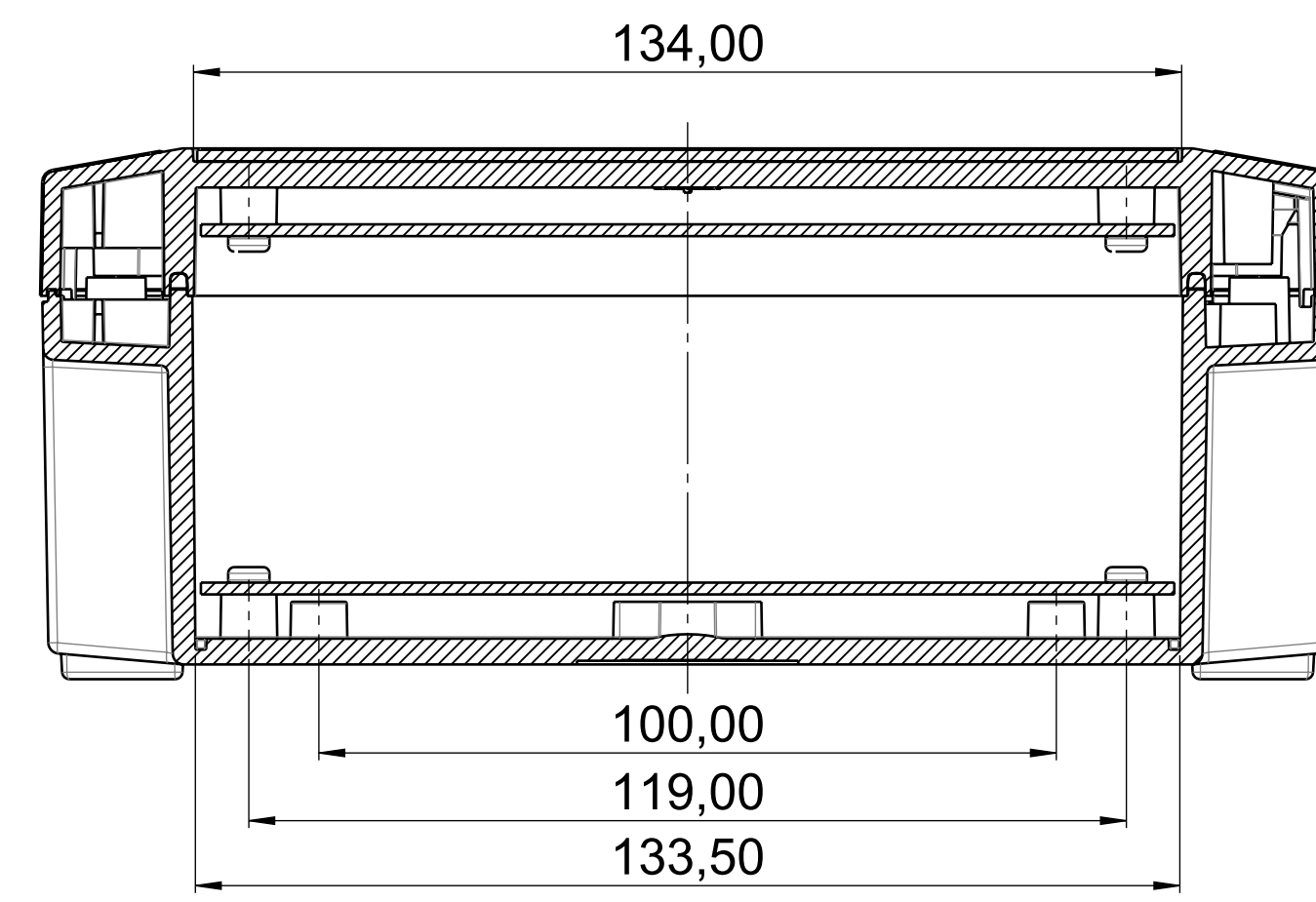
Schnitt A-A
