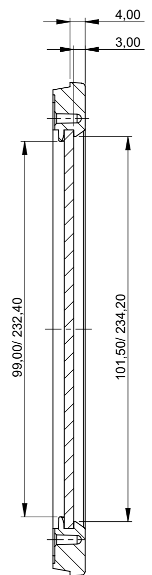
Schnitt A-A
