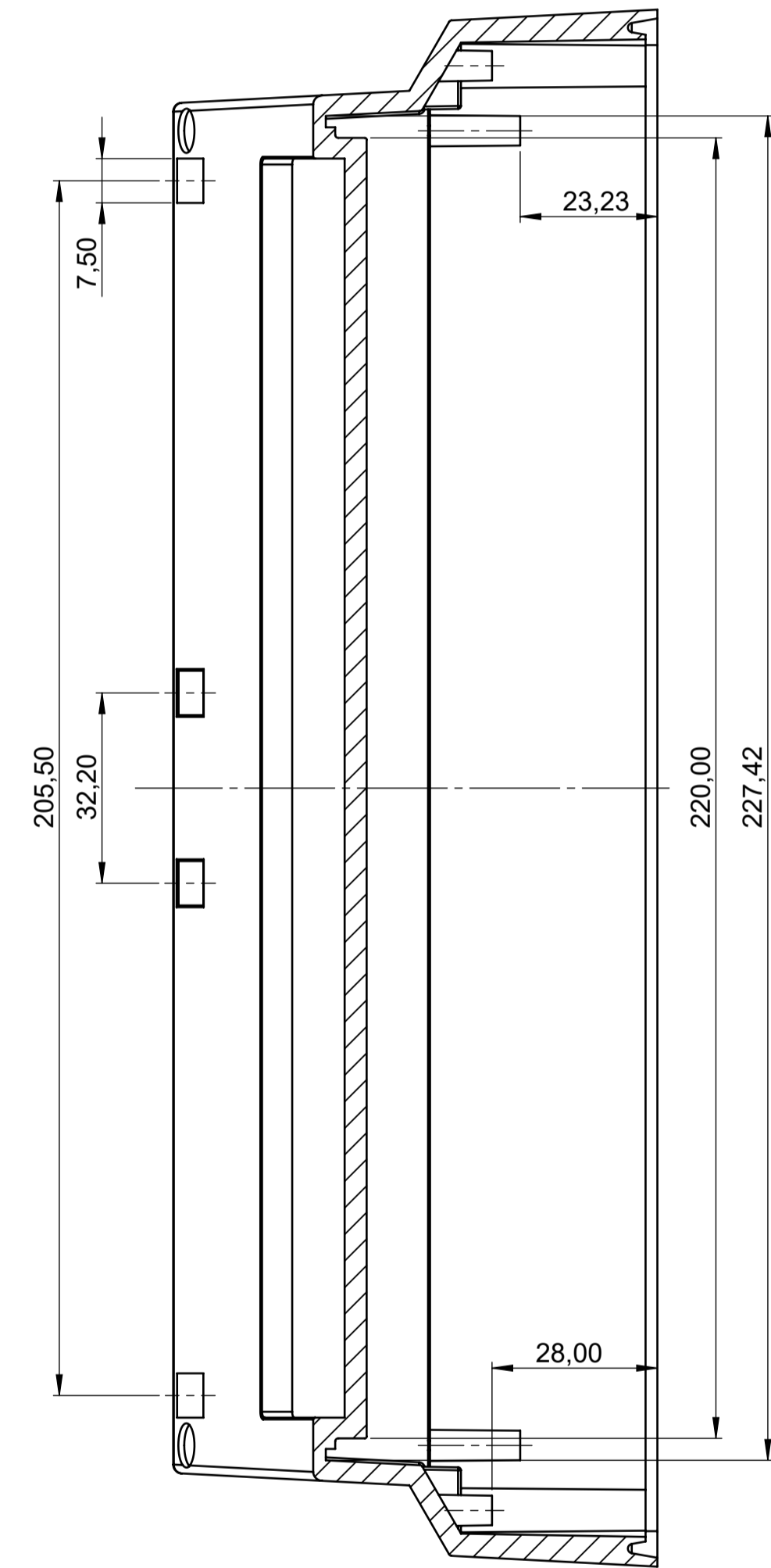
Schnitt A-A
