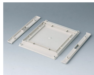
B4144257 Plaque inférieure avec réglettes à crans M ABS (UL 94 HB) gris blanc RAL 9002
