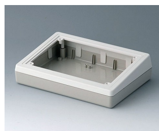
A9086265 BOITIER PUPITRE 190 F ABS (UL 94 HB) gris silex RAL 7032 190x138x47mm
