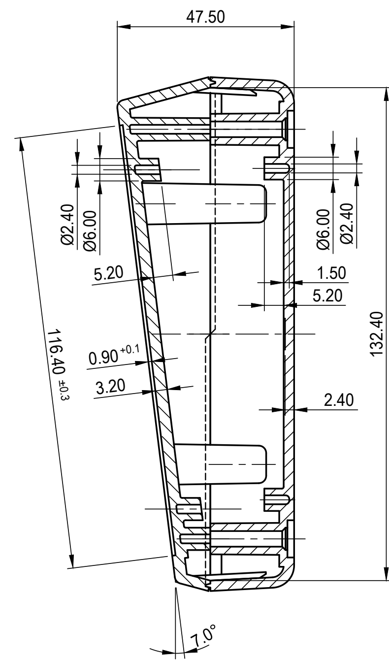
SCHNITT A-A section
