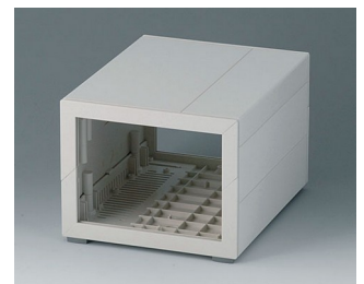
B2213217 MEDITEC E 160, ohne Griffbügel ABS (UL 94 HB) grauweiß RAL 9002 160x200x124mm IP 40
