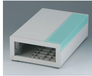
B2212005 MEDITEC E 220, ohne Griffbügel ABS (UL 94 HB) grauweiß RAL 9002 160x260x74mm IP 40
