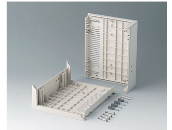
B2013107 L-Schalen E 160, m. Bohrung f. Griffb. ABS (UL 94 HB) grauweiß RAL 9002 160x200x74mm
