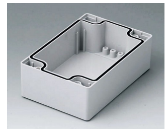
C2081202 Gehäuseschale 80, mit Dichtung PC (UL 94 HB) lichtgrau RAL 7035 120x80x40mm
