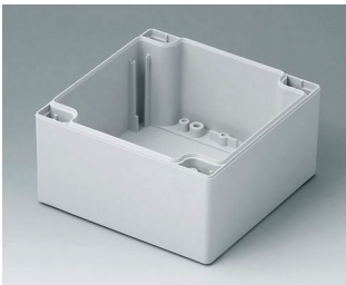
C2121202 Gehäuseschale 120, mit Feder PC (UL 94 HB) lichtgrau RAL 7035 120x120x60mm
